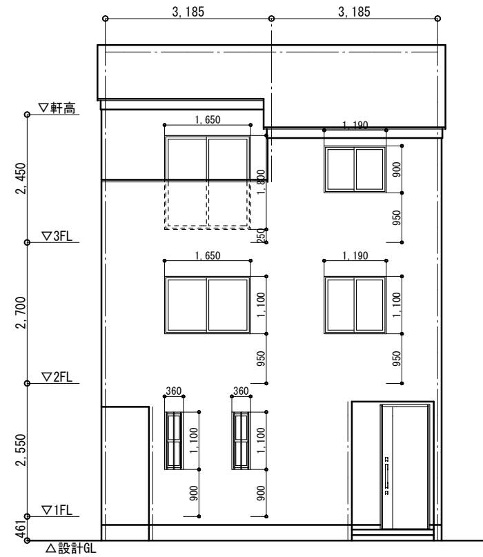
北面立面図 S=1:100
